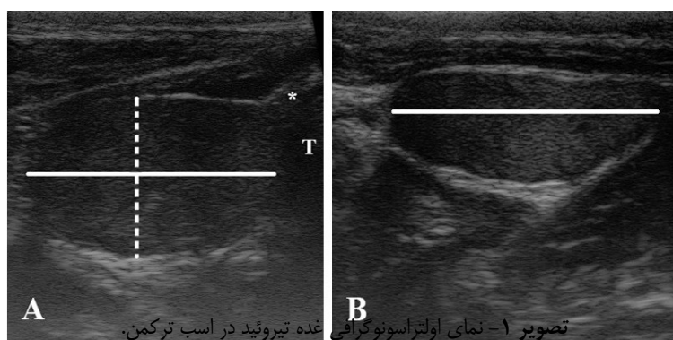
تصویر ۱- نمای اولتراسونوگرافی غده تیروئید در اسب ترکمن. A: نمای عرضی؛ خط ممتد (عرض لوب)، خط چین (ارتفاع لوب)، T (نای)، ستاره (عرض ایستموس) B: نمای طولی؛ خط ممتد نشان دهنده طول لوب تیروئید
