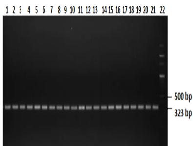
شکل ۴- الکتروفورز محصول PCR مربوط به تکثیر ژن iss (نمونه‌های مثبت ۳۲۳ جفت بازی)
